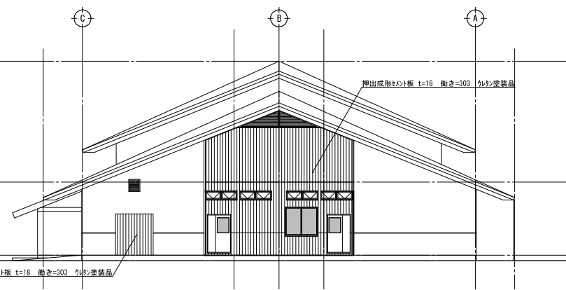
西側立面図 1/100 (1/200 A-3)
