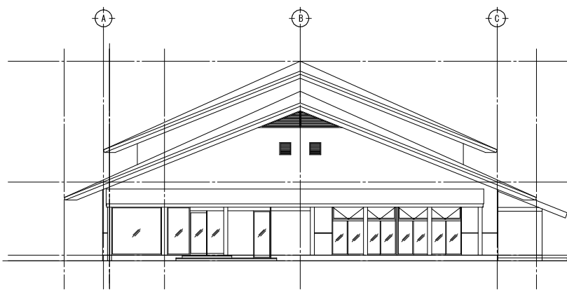
東側立面図 1/100 (1/200 A-3)
