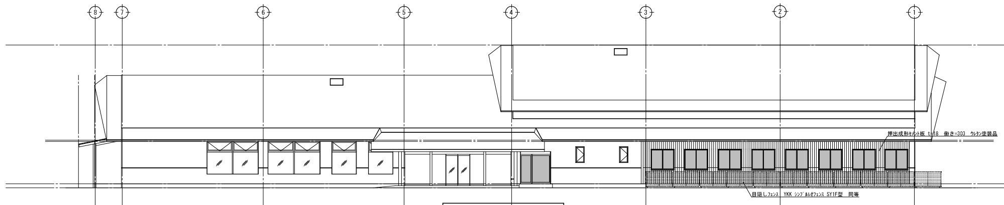
北側立面図 1/100 (1/200 A-3)
