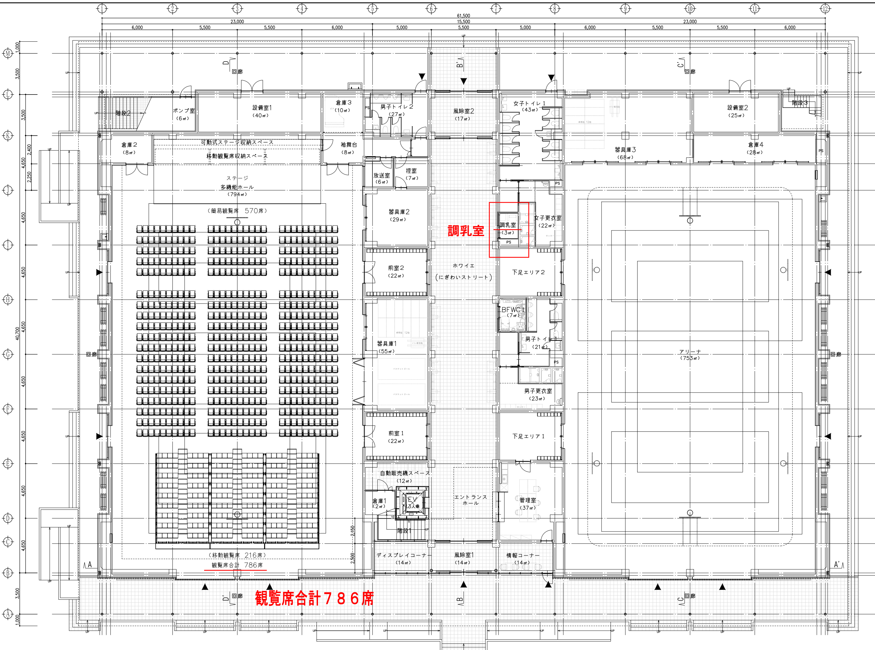
1階平面図 A3S-1/200
