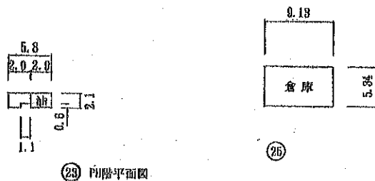
㉓ 1階平面図
