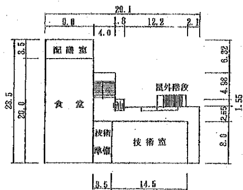
㉒ 1階平面図
