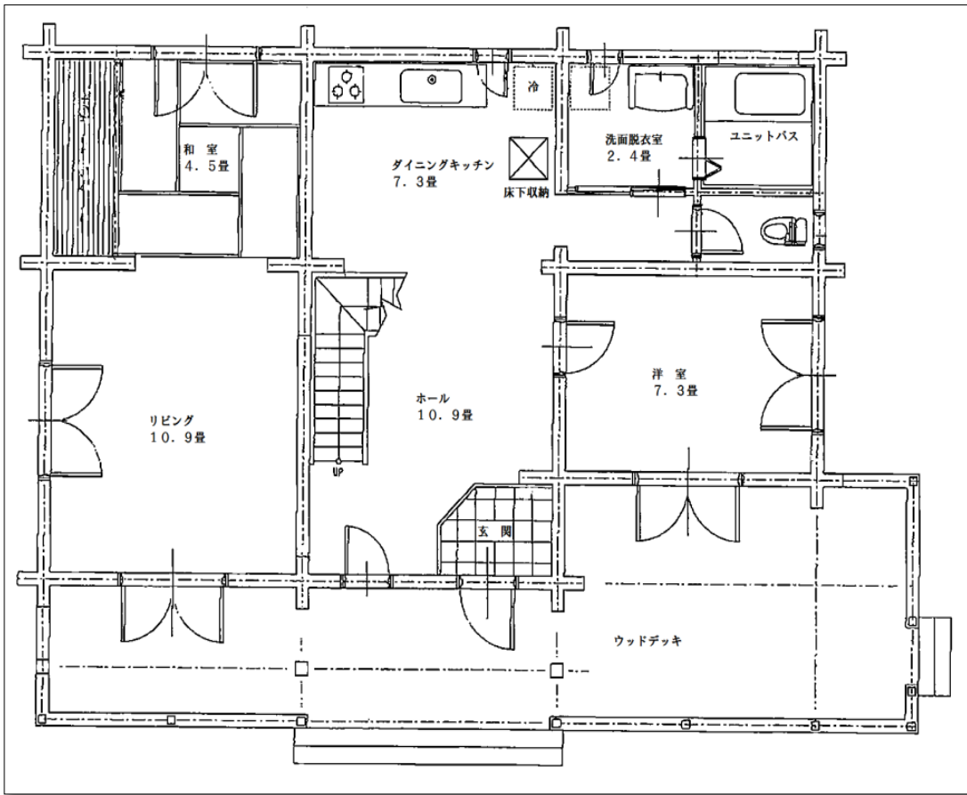
一階間取り図
